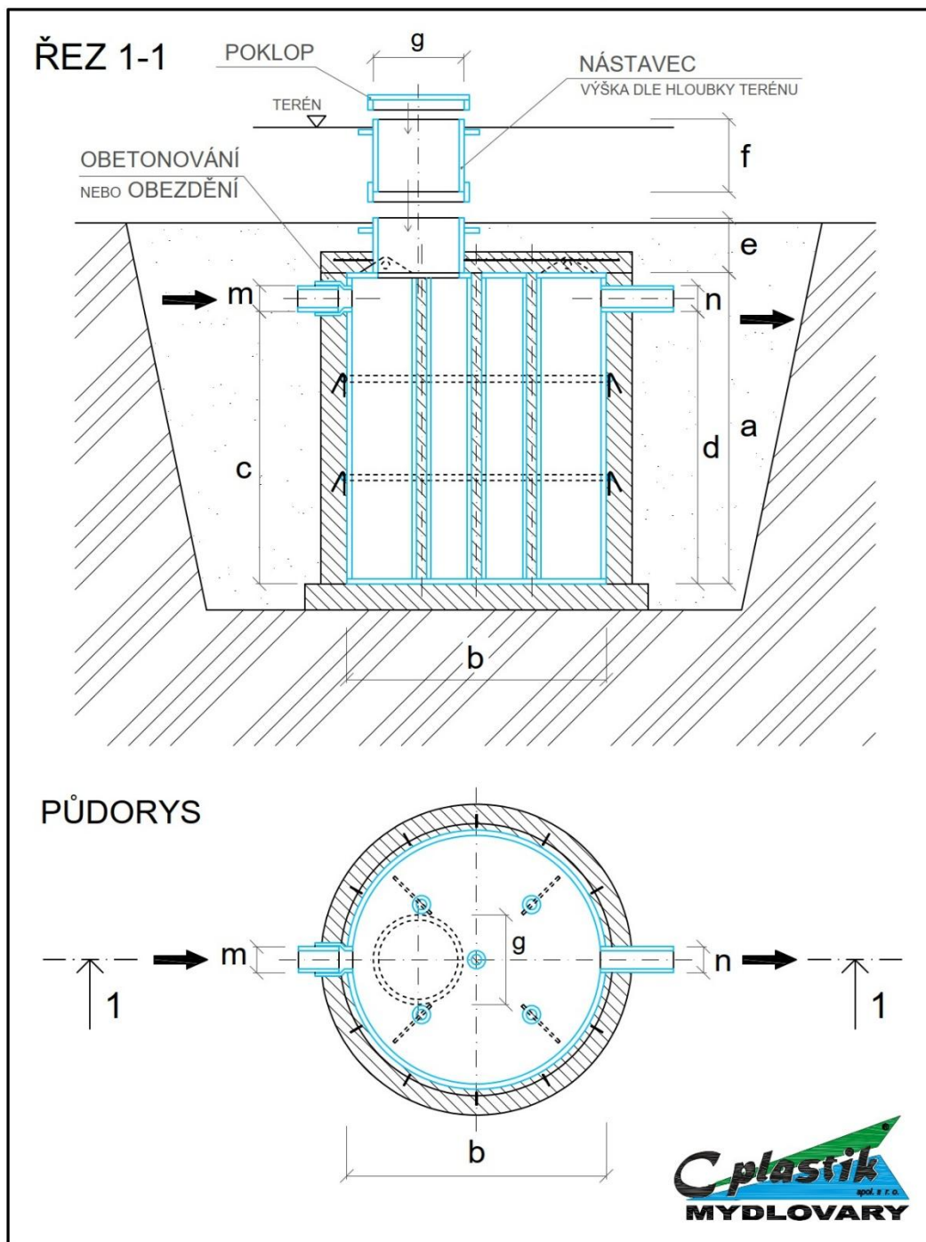
Retenční nádrž C VD 6 - rozměry v mm:
